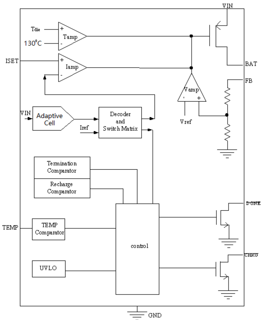
图 3 功能框图
